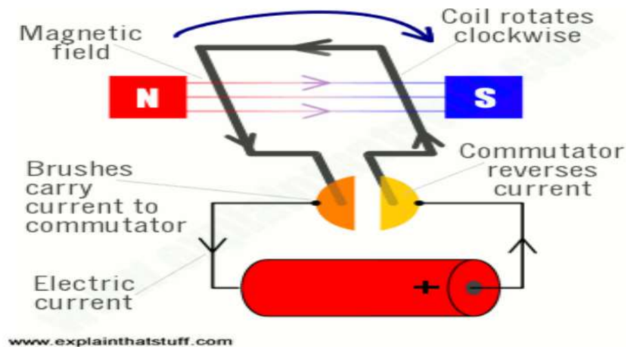
Fig:4.1.4a : DC Motor
