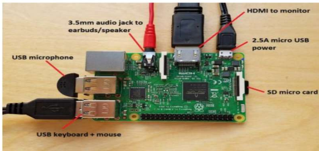
Fig : 4.1.1b : Raspberry pi board
