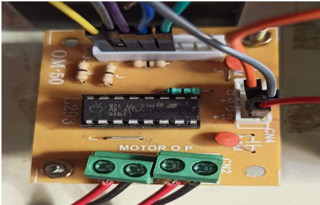
Fig: 4.1.5a : Driver IC
