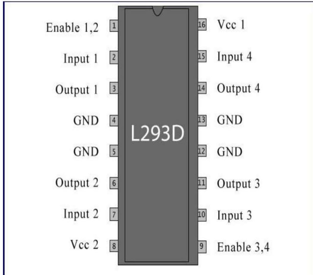
Fig: 4.1.5b : Pin Diagram
