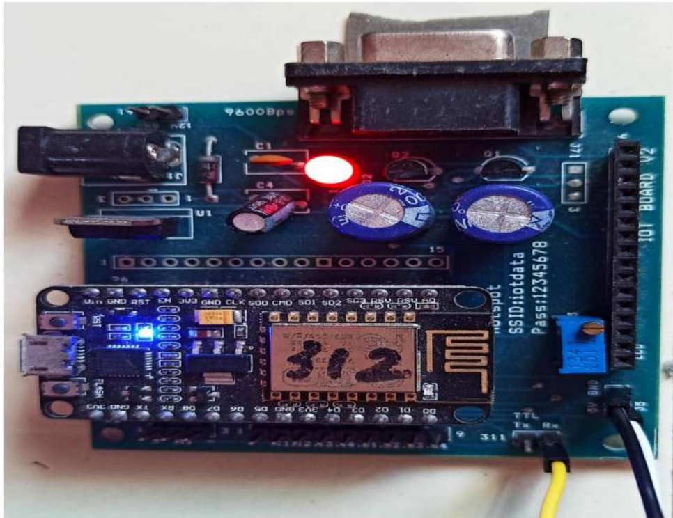
Fig: 4.1.6: ESP module
