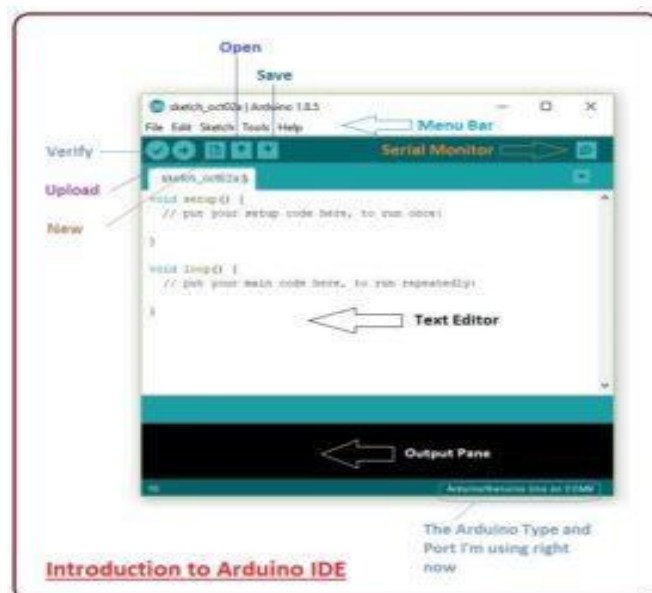
FIG 3.6 Arduino IDE
