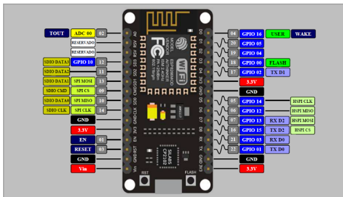
Fig 3.1 NodeMCU
