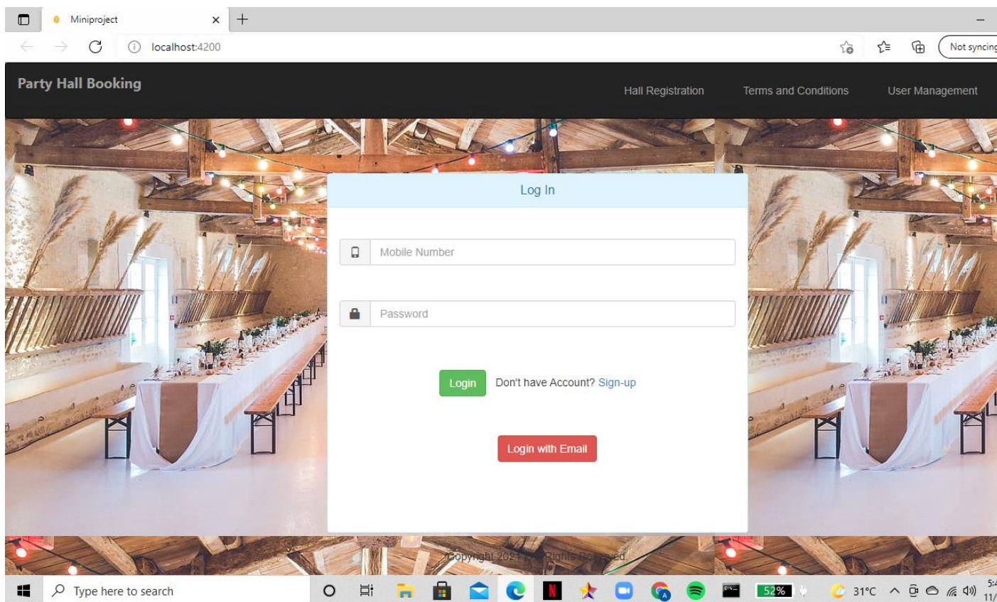
Fig.1.1 : Login Page
