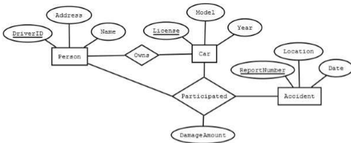
Fig.2. ER diagram
