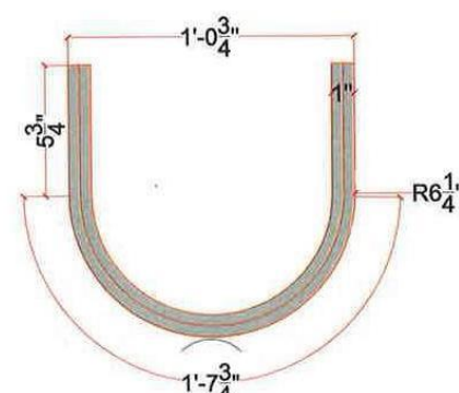
DETAIL A1
