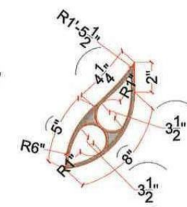
DETAIL A5
