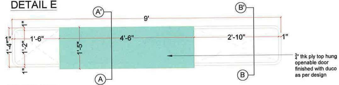
ELEVATION
