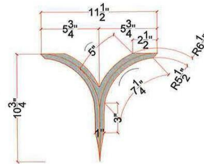
DETAIL A2
