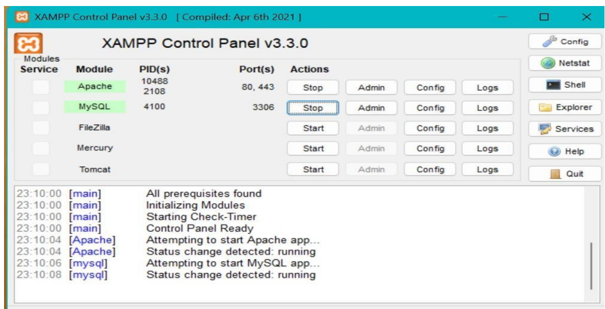
Fig-3:Open Xampp
