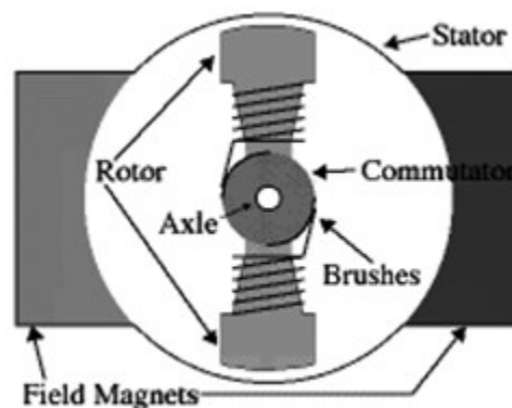
Fig:4.11 Dc Motor
