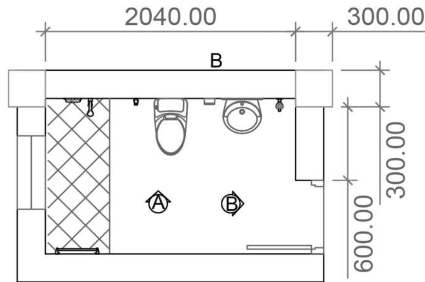
TOILET LAYOUT
