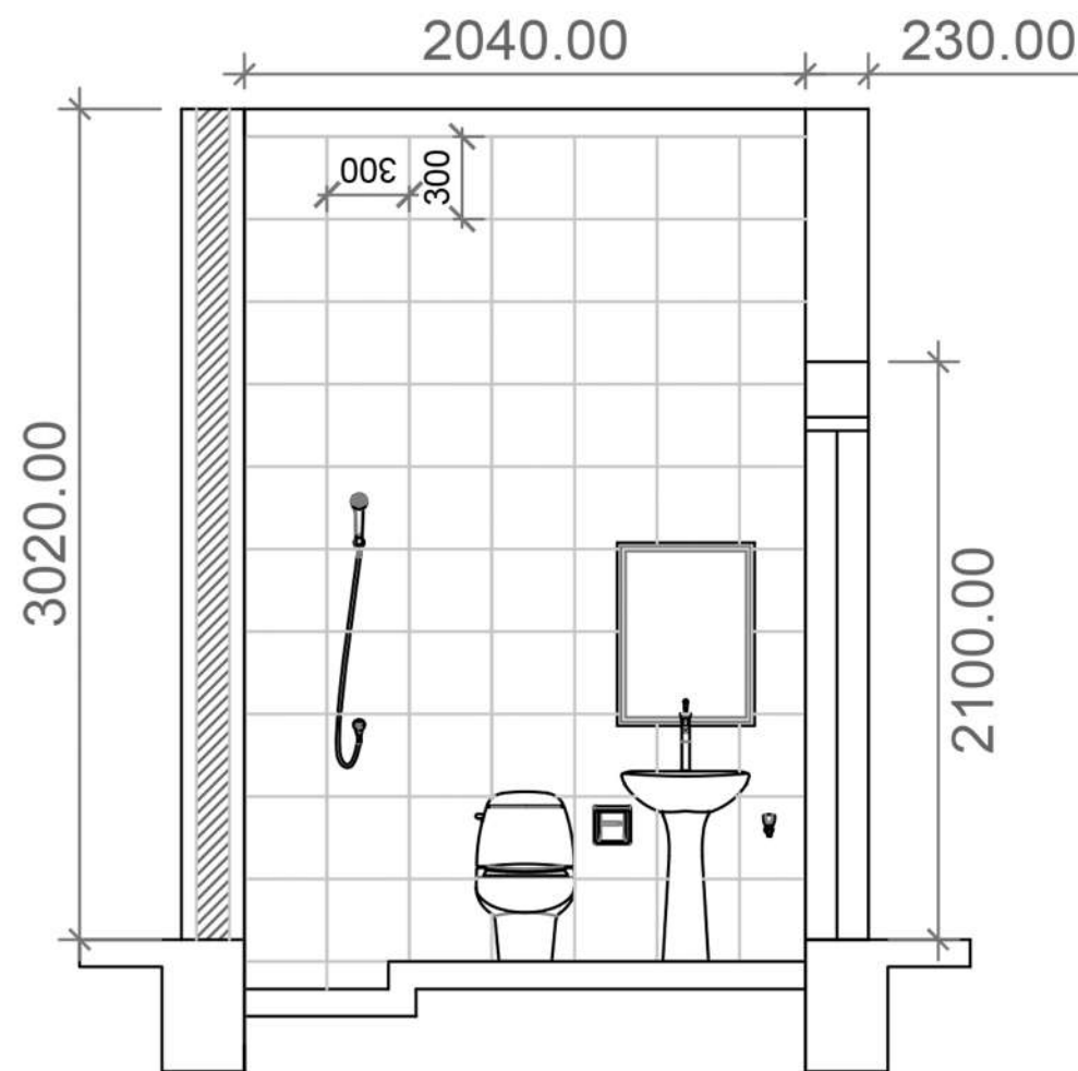
ELEVATION -A
