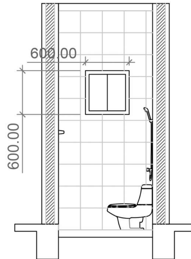
ELEVATION -B
