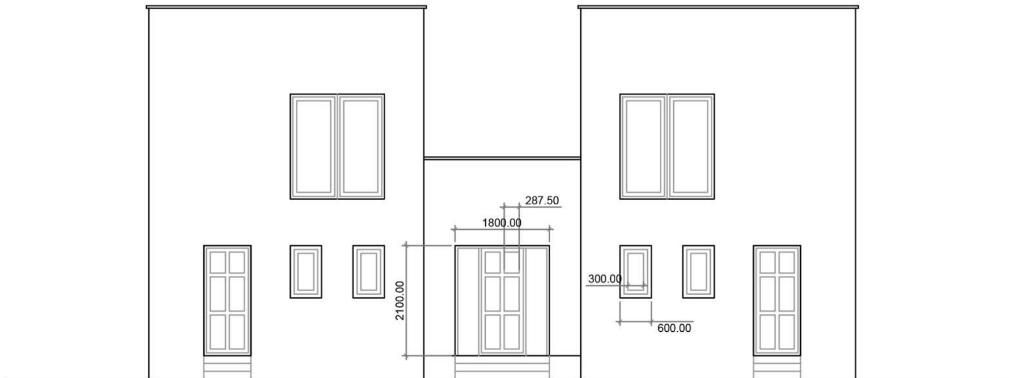
ELEVATION
