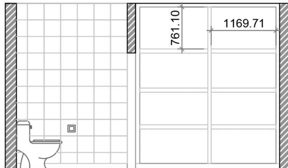
ELEVATION -B
