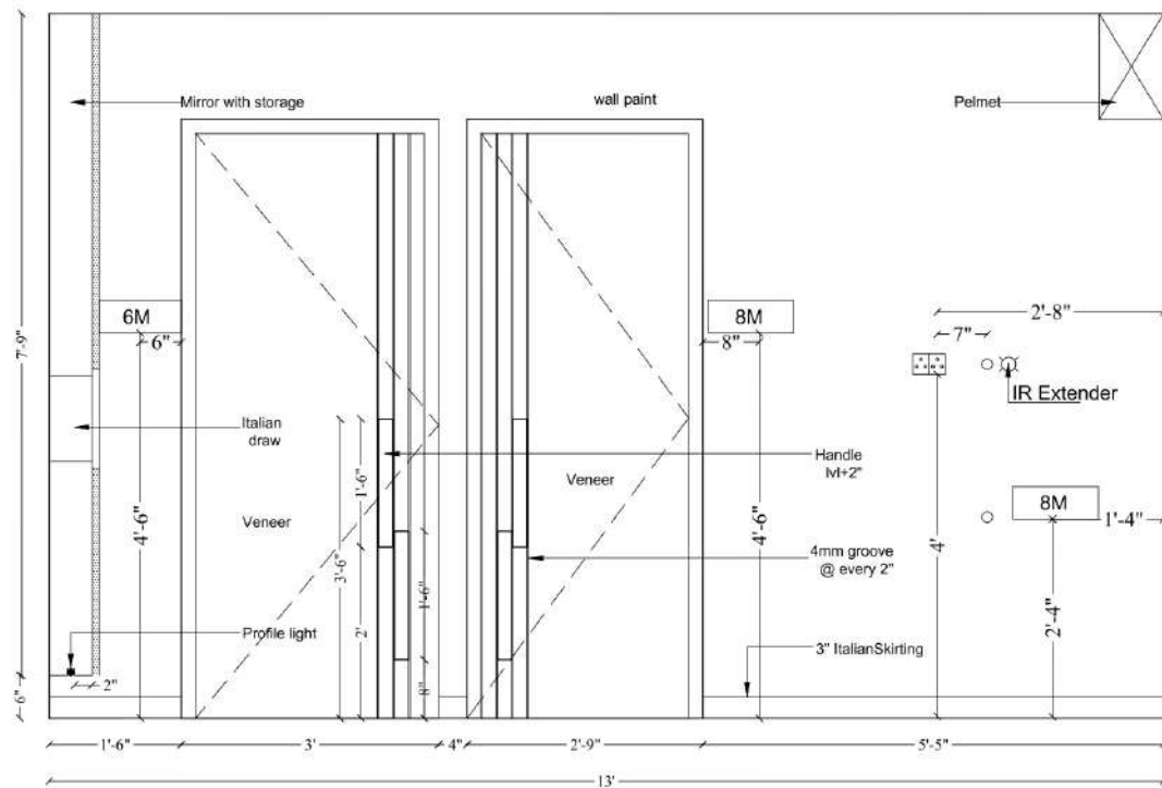
Elevation B
