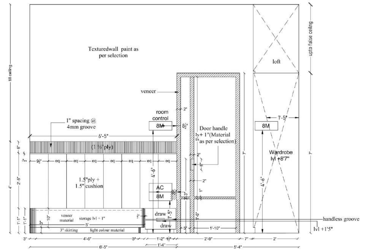
Elevation-A
