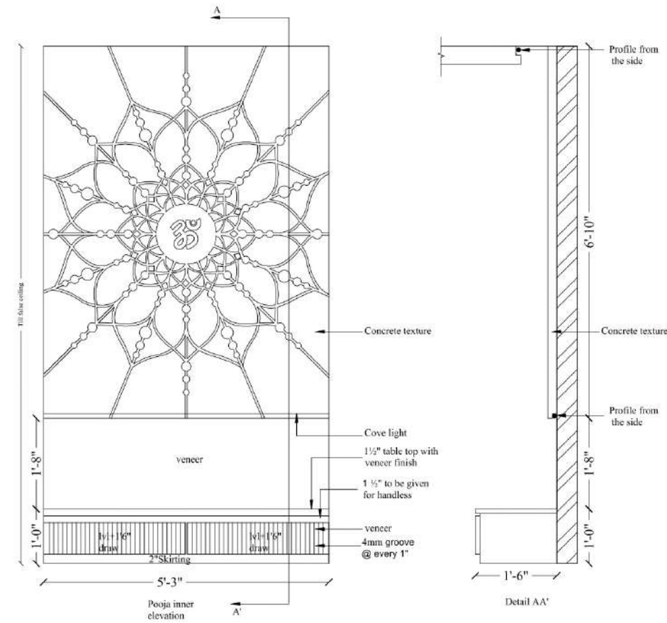
Elevation-A
