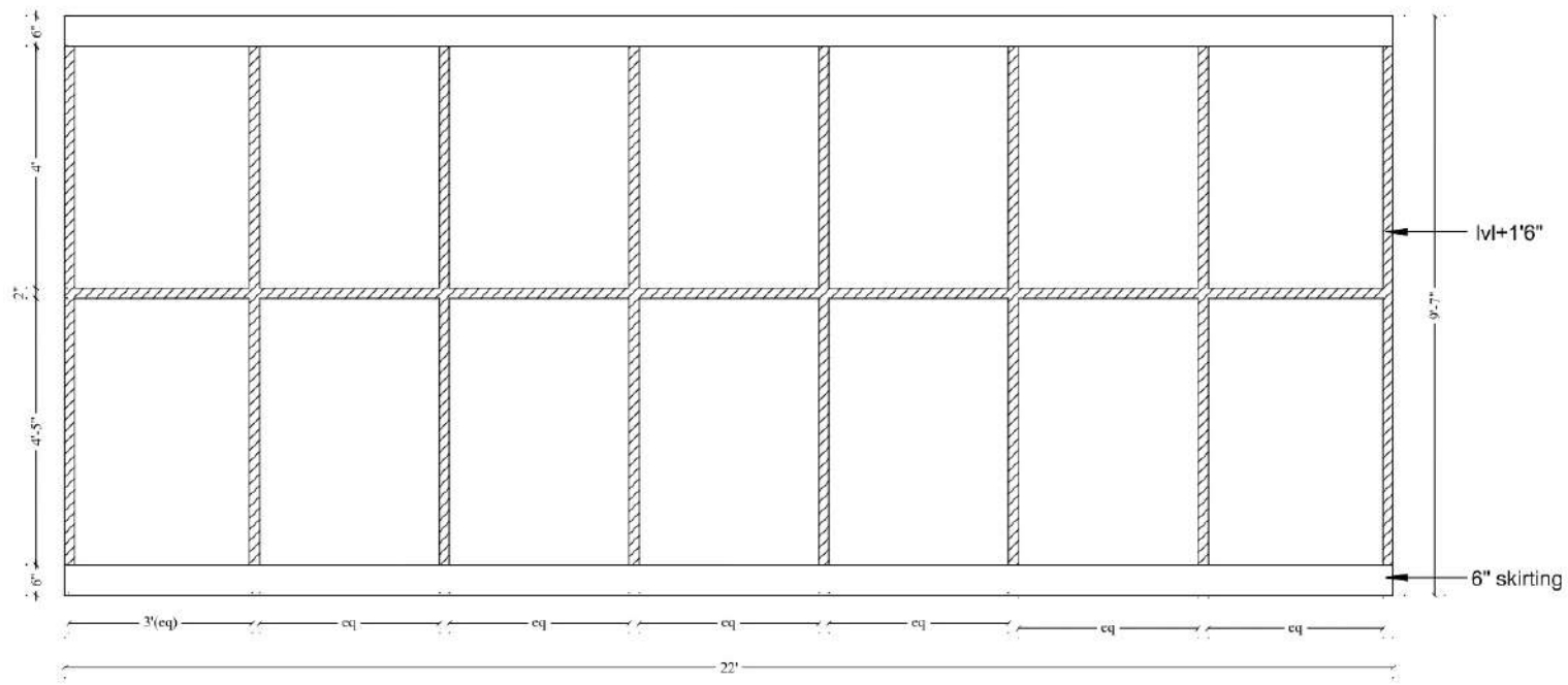
Elevation B
