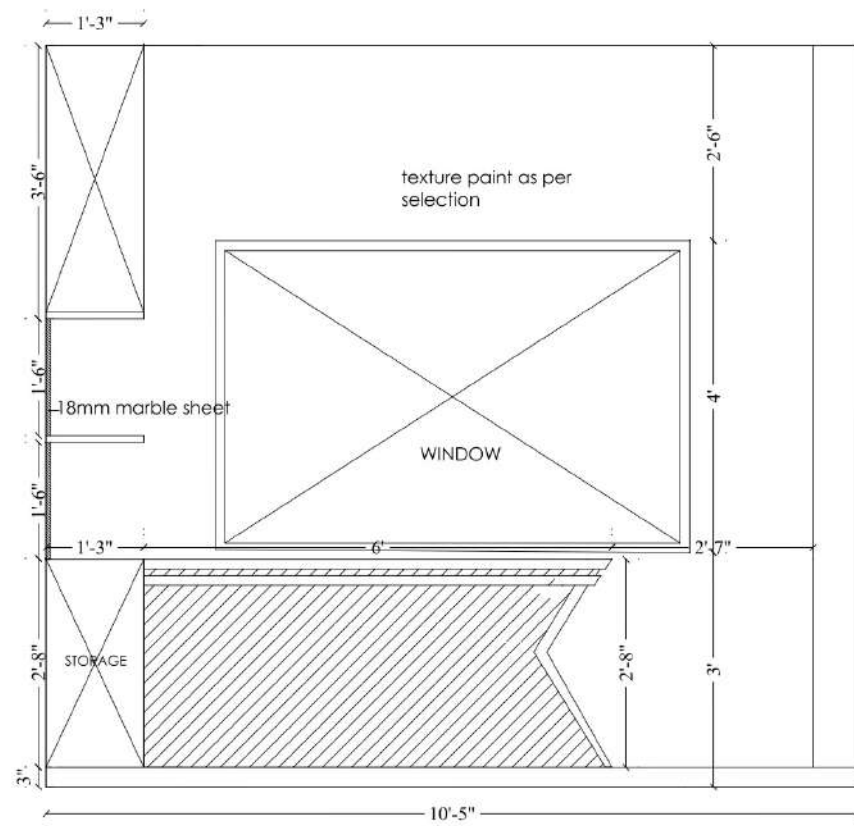
Elevation B
