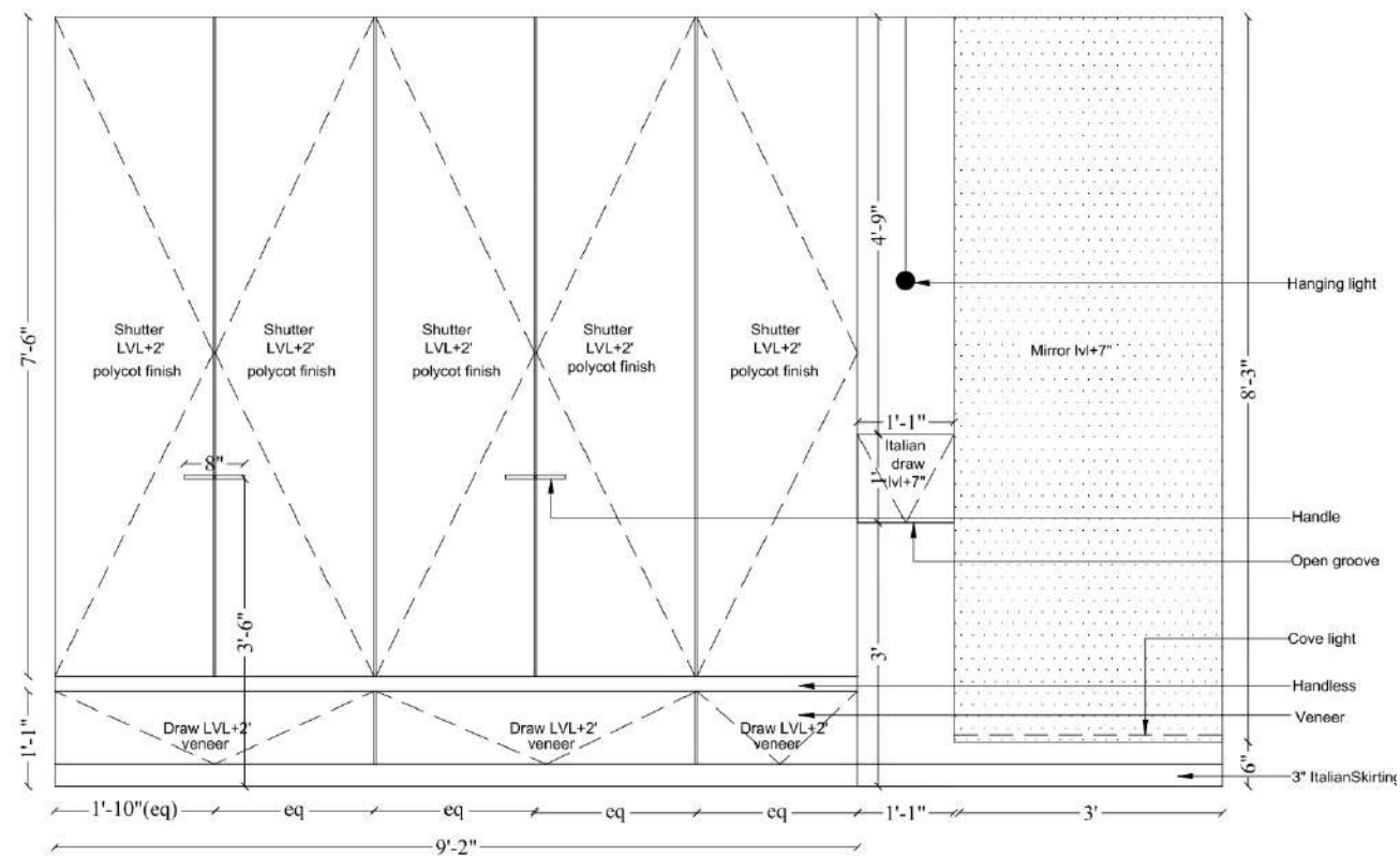
Elevation A
