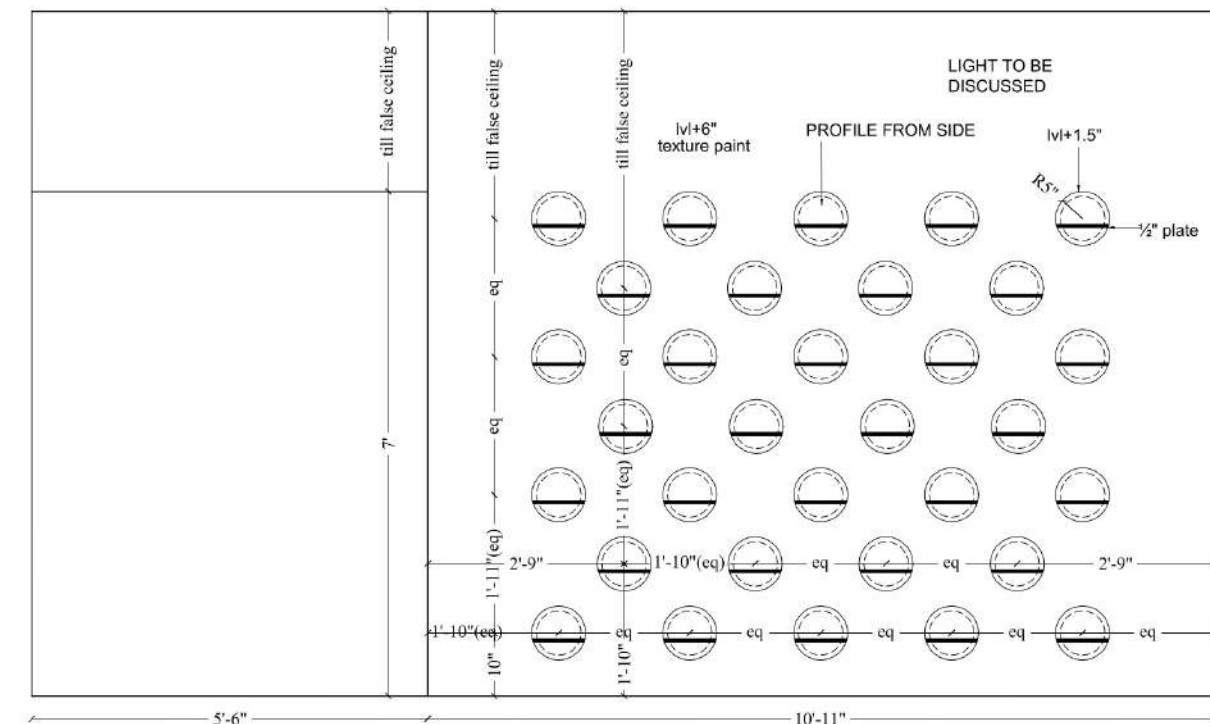
Elevation A
