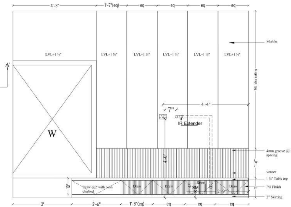
Elevation-A
