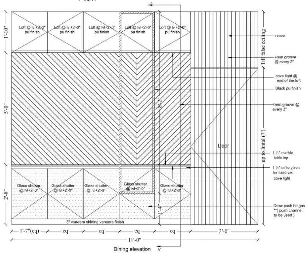
Elevation-A
