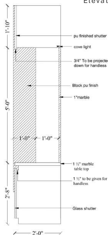
Elevation-A
