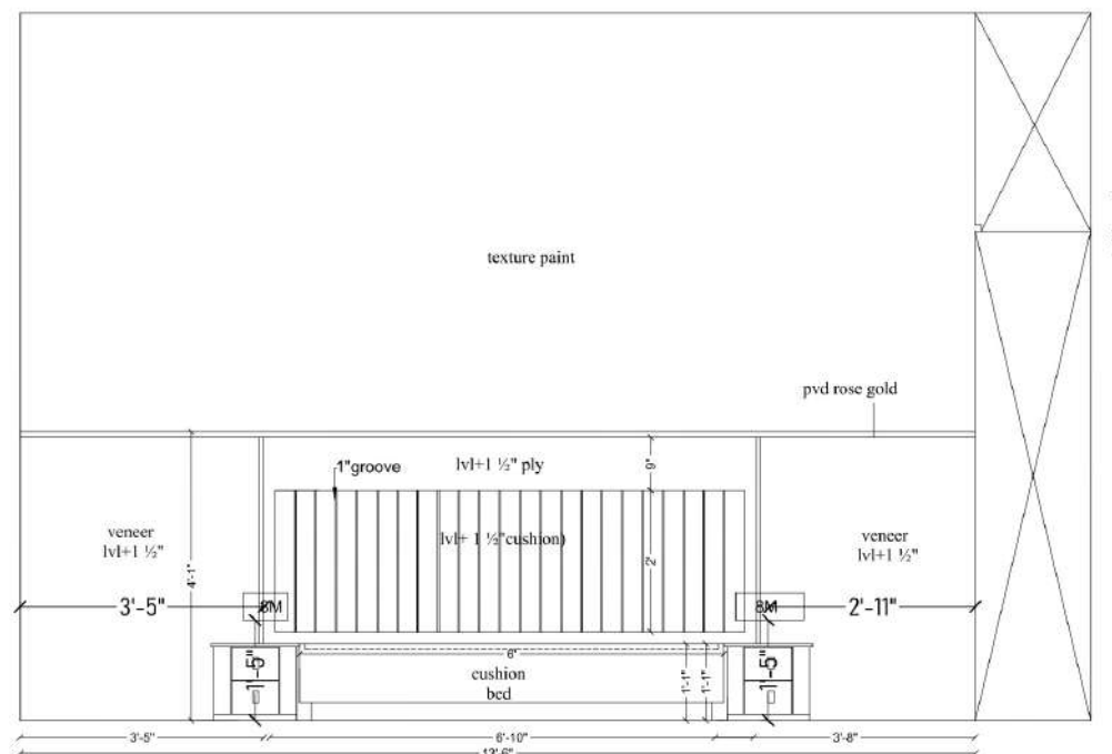
Elevation-A
