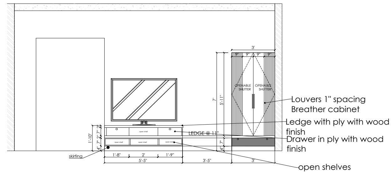
ELEVATION B
