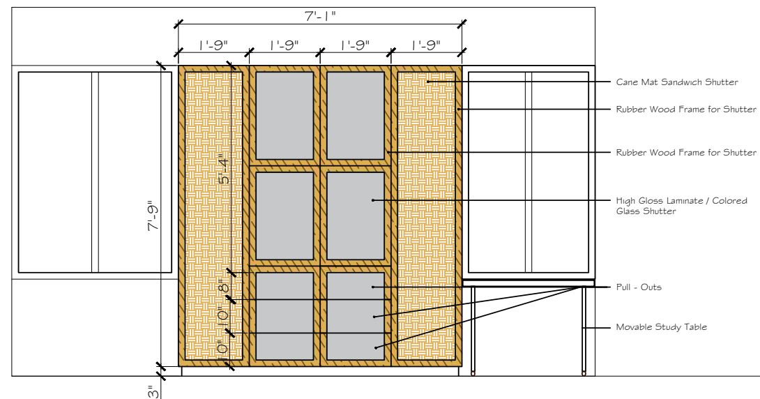
ELEVATION
