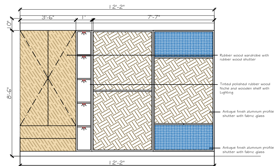
ELEVATION B
