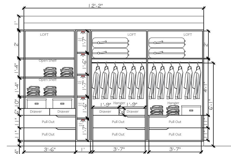
INTERIORS
