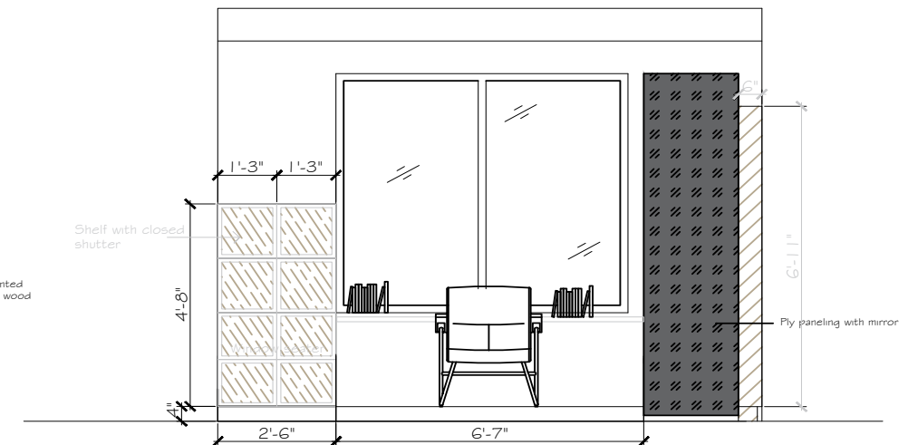
ELEVATION A
