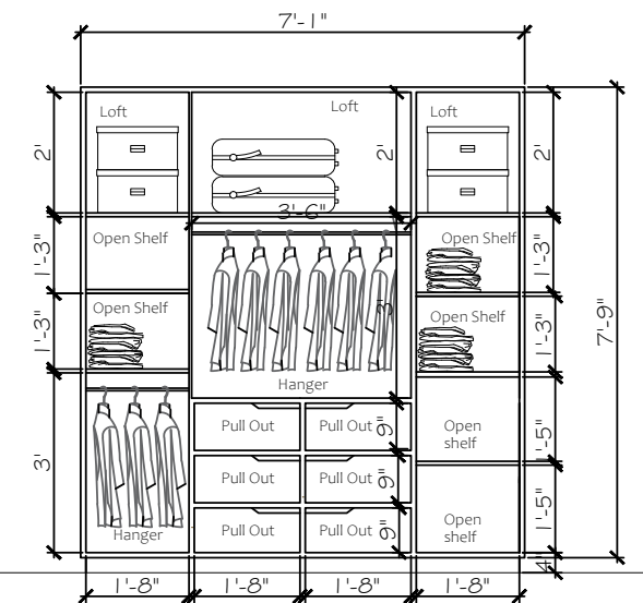
INTERIORS
