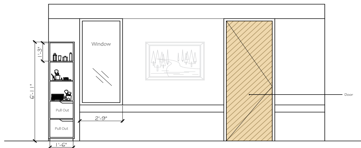
ELEVATION B
