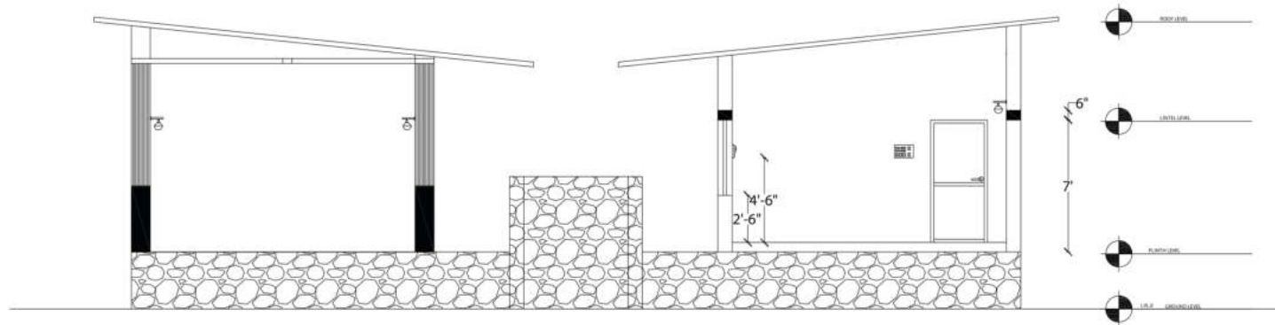
SECTION - AB
