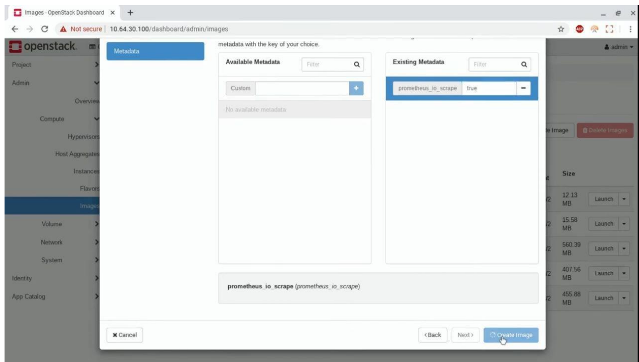
FIG.3.3.3 Metadata
