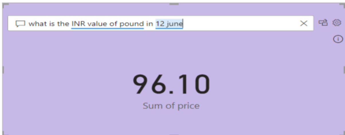
FIGURE 6.2 : Q&A
