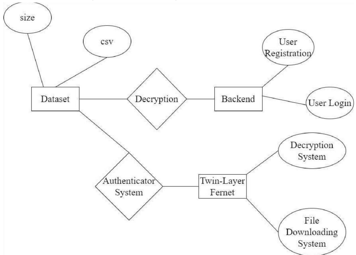
Fig 3.8 – ER Diagram
