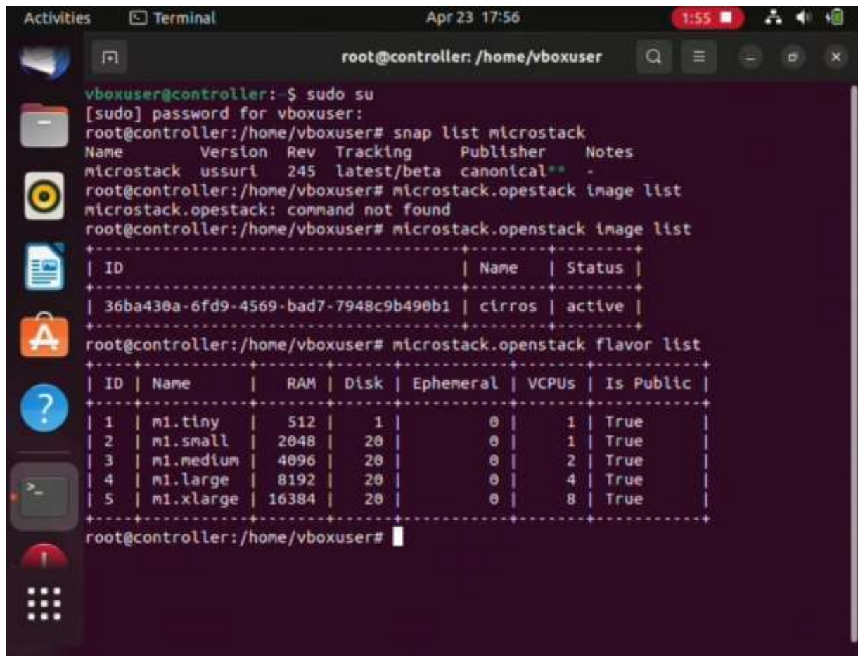
Fig 6.2: Vboxuser Login
