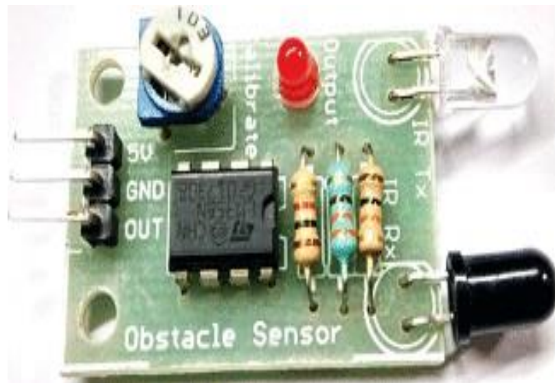
Fig 4.8: IR Sensor
