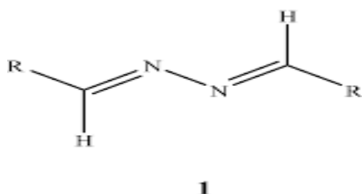
Fig:1.1.a: 2,3 diaza
