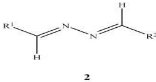
Fig:1.1.b: 1,3 butadiene
