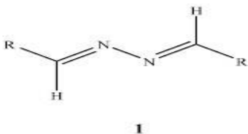
Fig:1.1.a: 2,3 diaza
