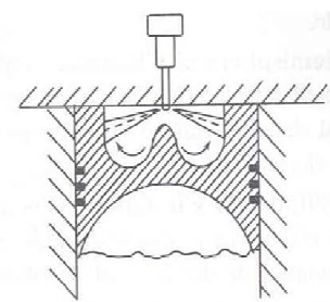
(d) Toroidal chamber
