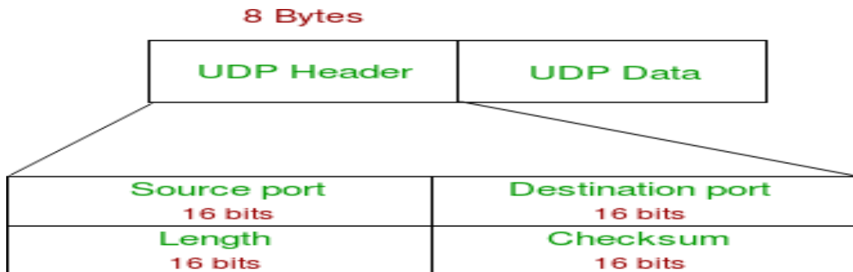
Fig 3.5:UDP Header
