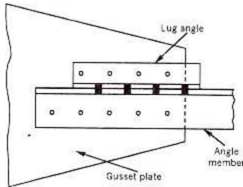
Fig 7 Lug Angle
