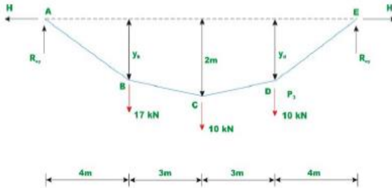
Fig. 31.4 Example 31.1
