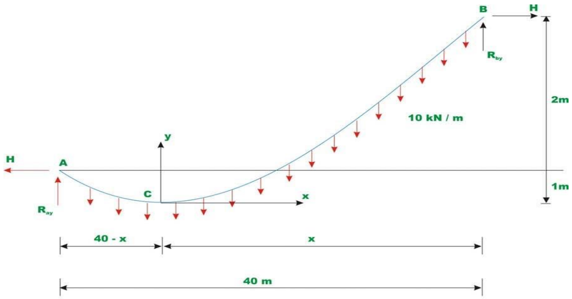
Fig. 31.5 Example 31.2
